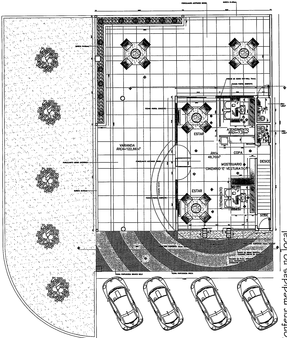
LAYOUT TÉRREO Escala: 1/50
