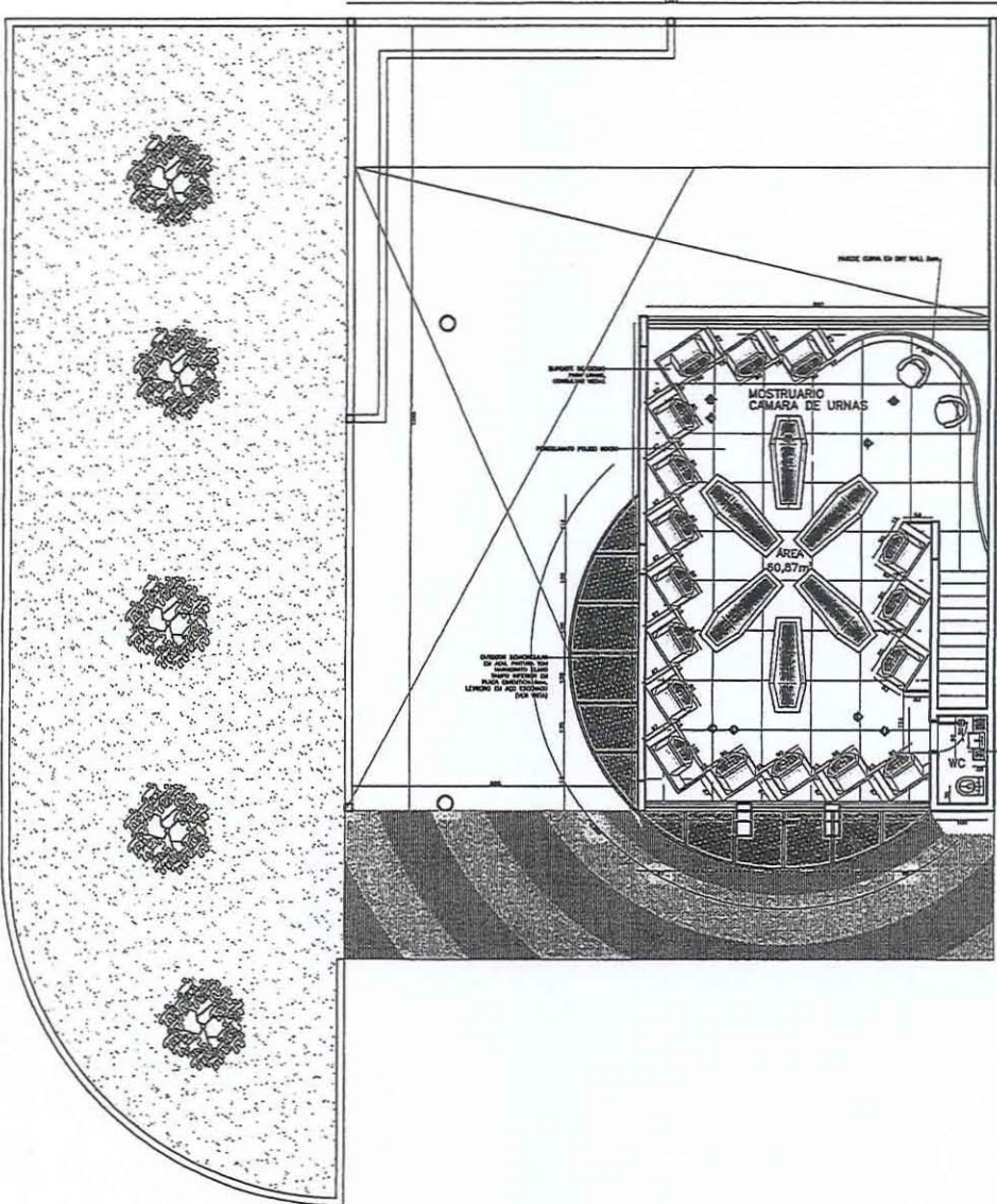
LAYOUT SUPERIOR Escala 1:100
